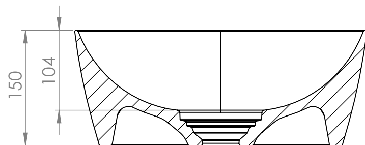
SECCIÓN A-A ESCALA 1 : 5
