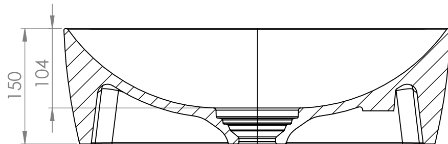
SECCIÓN A-A ESCALA 1 : 5
